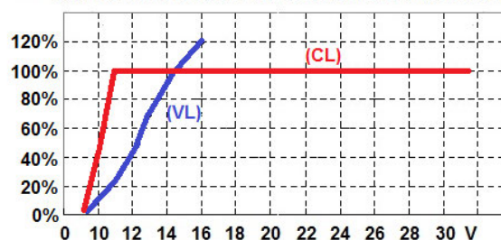
Luminosità in funzione della Tensione di alimentazione
